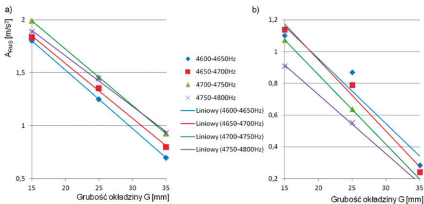
Rys. 8. Zależność wartości skutecznej przyspieszeń drgań ARMS od grubości okładzin czernych: a) dla tarczy typu 590x110, pomiar drgań w kierunku Y_1 , b) dla tarczy typu 590x110, pomiar drgań w kierunku Y_2
