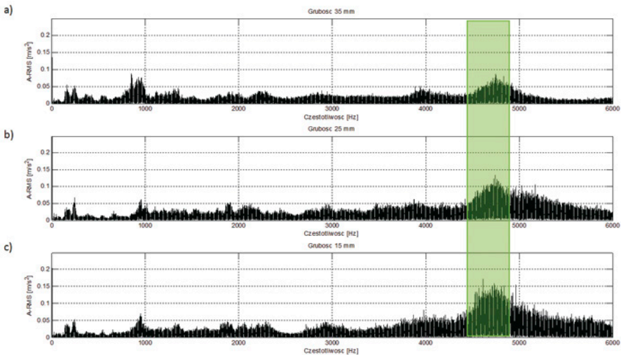
Rys. 4. Zależność amplitudy przyspieszeń drgań od częstotliwości dla różnych grubości okładziny przy hamowaniu ze stałą mocą na tarczy typu 590×110, dla kierunku Y_z ; a) grubość okładziny G1=35 mm, b) grubość okładziny G2=25 mm, c) grubość okładziny G3=15 mm
