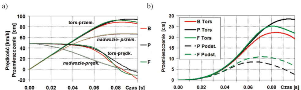
Rys. 14. Kinematyka manekina w testach B, P i F; a) prędkość i przemieszczenie nadwozia i torsu względem podłoża b) przemieszczenie torsu i podstawki względem podłogi nadwozia
