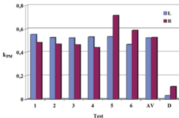
Rys. 7. Współczynnik zmniejszania emisji cząstek stałych - k_{PM} z tarczowego układu hamulcowego samochodu w poszczególnych badaniach, AV - wartość średnia współczynnika oraz D - odchylenie standardowe współczynnika, L - lewa strona samochodu, R - prawa strona samochodu
