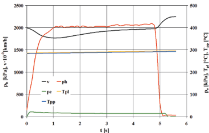
Rys. 6. Przykład przebiegów prędkości samochodu - v, ciśnienia w układzie hamulcowym - p_h , podciśnienia w układzie pneumatycznym - p_e oraz temperatur tarcz hamulców: lewej - T_{pi} i prawej - T_{pp} podczas hamowania samochodu w specjalnym teście jezdnych
