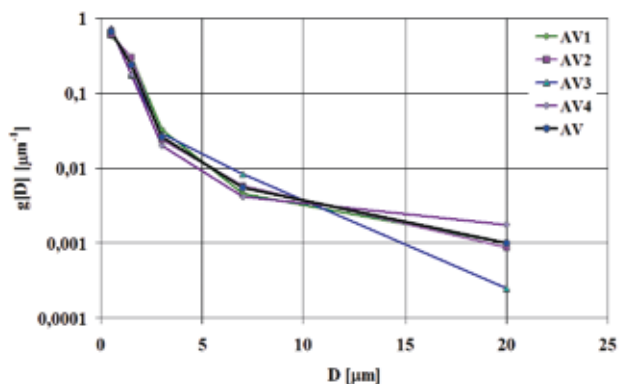
Rys. 10. Gęstość prawdopodobieństwa średnicy zastępczej cząstek pyłów próbki z hamulca tarczowego: wartości średnie dla poszczególnych miejsc analizy AV1 – AV4 oraz wartość średnia dla próbki – AV
