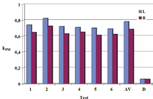
Rys. 8. Współczynnik zmniejszania emisji cząstek stałych - k_{PM} z bębnowego układu hamulcowego samochodu w poszczególnych badaniach, AV - wartość średnia współczynnika oraz D - odchylenie standardowe współczynnika, L - lewa strona samochodu, R - prawa strona samochodu
