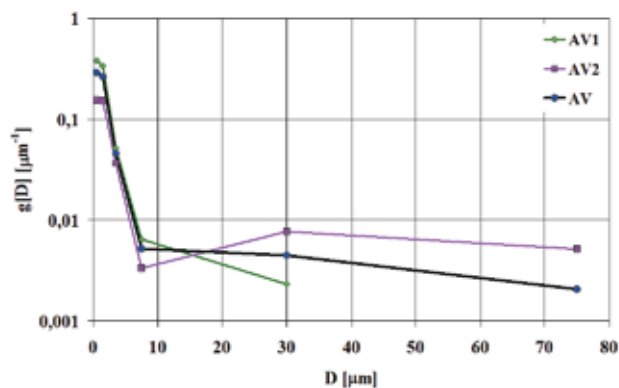
Rys. 11. Gęstość prawdopodobieństwa średnicy zastępczej cząstek pyłów próbki z hamulca bębnowego: wartości średnie dla poszczególnych miejsc analizy – AV1 i AV2 oraz wartość średnia dla całej próbki – AV
