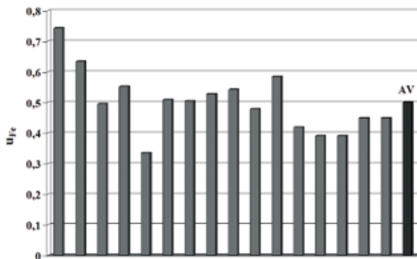
Rys. 12. Udział pola powierzchni przekroju ziaren żelaza – u_{Fe} w cząstkach stałych z tarczowego układu hamulcowego: AV – wartość średnia
