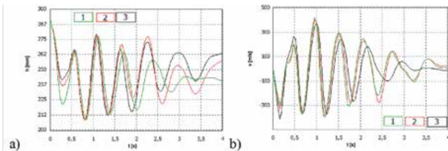
Rys. 4. Wartości a) przemieszczenia i b) prędkości końców amortyzatora w funkcji czasu dla trzech sposobów hamowania. 1 – z użyciem systemu ABS system, 2 – hamowanie pulsacyjne, 3 – hamowanie z blokowaniem kół
