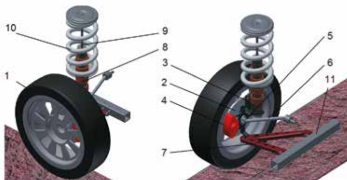
Rys. 2. Kolumna McPhersona stanowiąca układ dynamiczny o dwóch stopniach swobody; 1 - koło, 2 - tarcza hamulcowa, 3 - zwrotnica, 4 - zacisk, 5 - przegub, 6 - półoś napędowa, 7 - wahacz, 8 - stojan silnika (cylinder amortyzatora), 9 - tłoczysko z magnesami, 10 - sprężyna resorowa, 11 - karoseria samochodu
