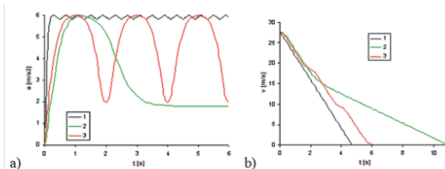
Rys. 3. Wartości a) opóźnień i b) prędkości samochodu w funkcji czasu dla trzech sposobów hamowania. 1 – z użyciem systemu ABS system, 2 – hamowanie pulsacyjne, 3 – hamowanie z blokowaniem kół
