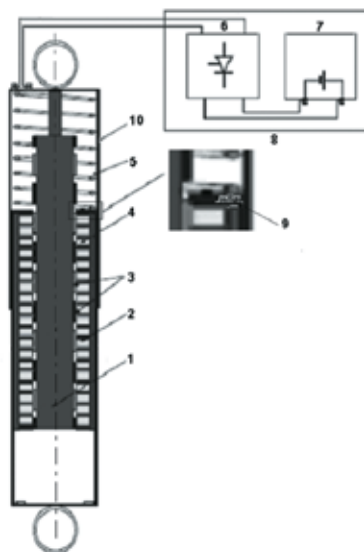
Rys. 1. Amortyzator elektromagnetyczny; 1 - tłok z magnesami trwałymi, 2 - cylinder z układem cewek, 3 - magnesy stałe, 4 - cewka, 5 - wydrążona sprężyna z umieszczonymi wewnątrz przewodami elektrycznymi, 6 - sterowany prostownik, 7 - akumulator, 8 - zespół magazynowania energii, 9 - zaciski przewodów, 10 - pokrywa
