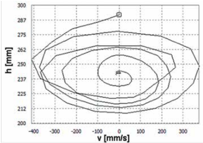
Rys. 5. Wykres fazowy dla końców amortyzatora podczas hamowania z działaniem systemu ABS
